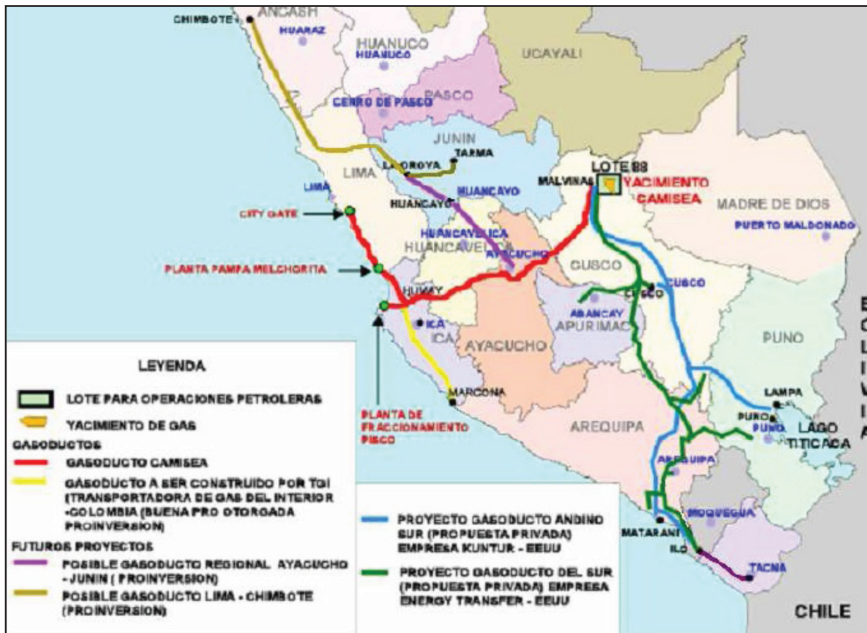
Gráfico N° 21 Interconexión macrorregional por el gas de Kamisea
