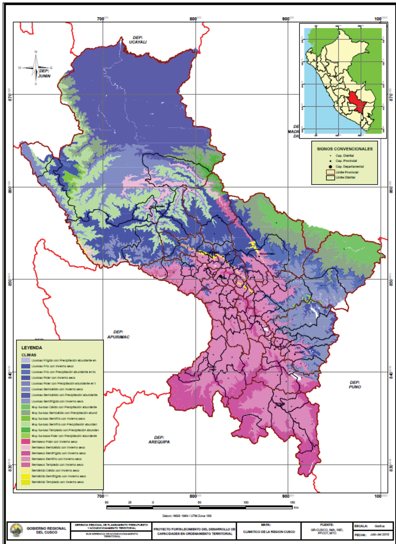
Mapa N° 08 Climas del Departamento
