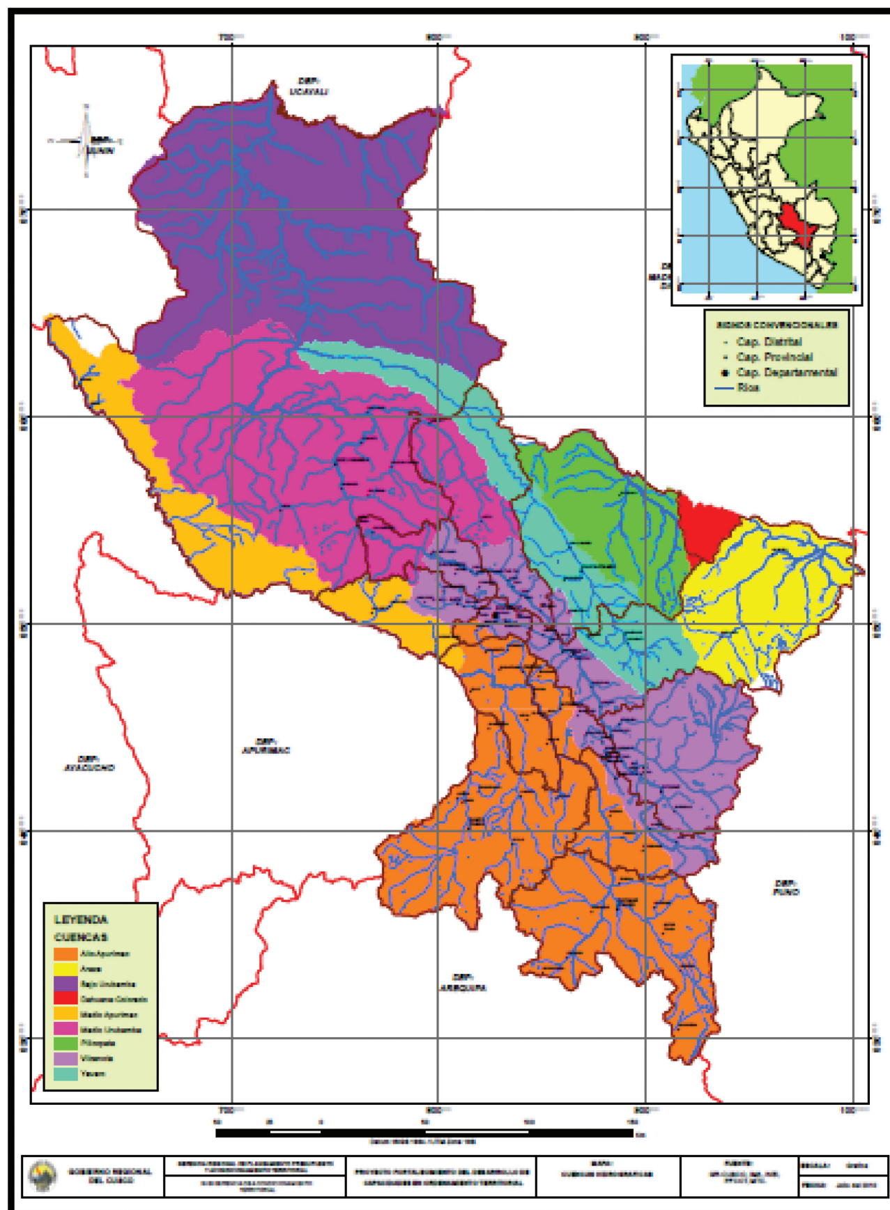
Mapa N° 09 Cuencas y Subcuencas
